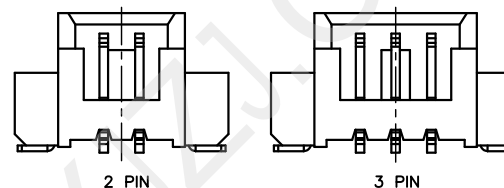
LOCK CONFIGURATION (锁扣位置)
