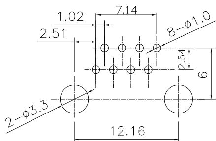
PCB参考图
