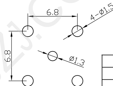
PCB板
