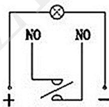
电器原理图
