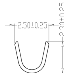
SEC:B-B
